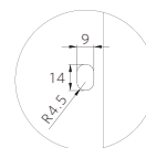
I 部取付固定穴拡大図
