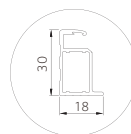
B-B 断面図
