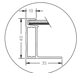
A-A 断面図
